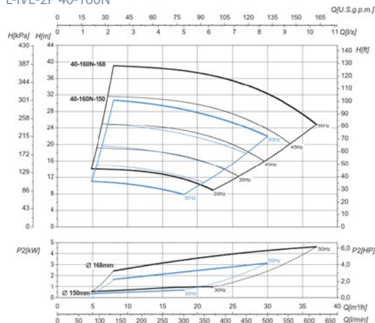
L-IVE-2P 40-160N
