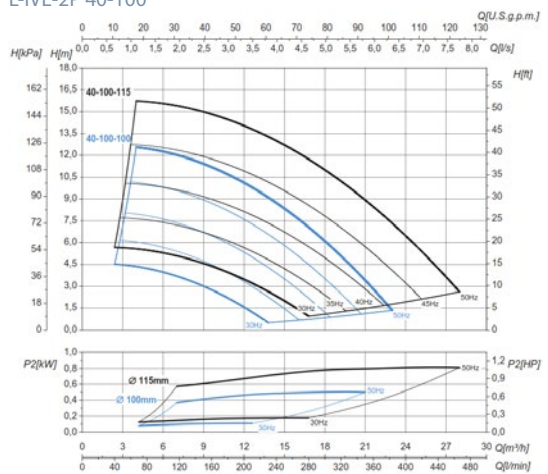
L-IVE-2P 40-100
