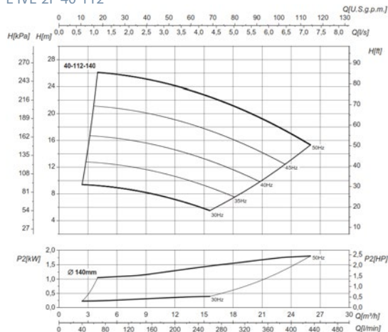
L-IVE-2P 40-112
