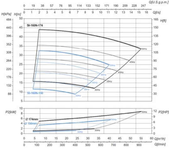
L-IVE-2P 50-160N
