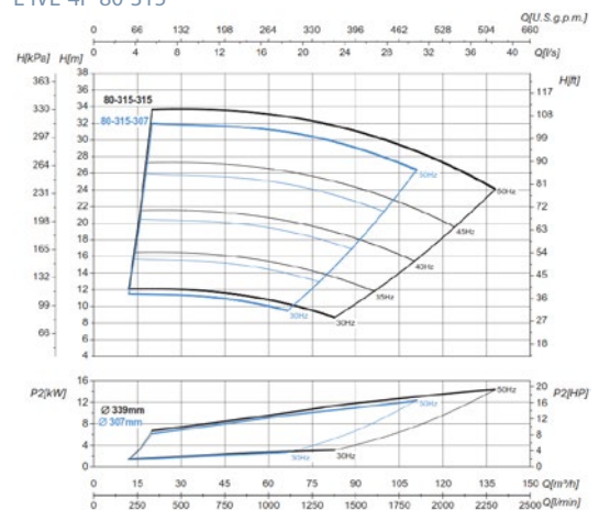
L-IVE-4P-80-315
