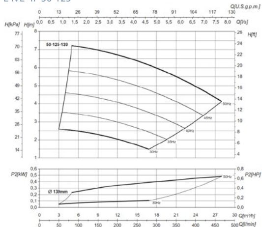
L-IVE-4P 50-12S
