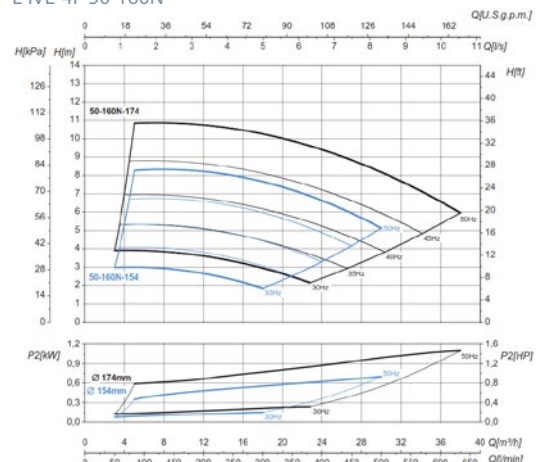
L-IVE-4P 50-160N
