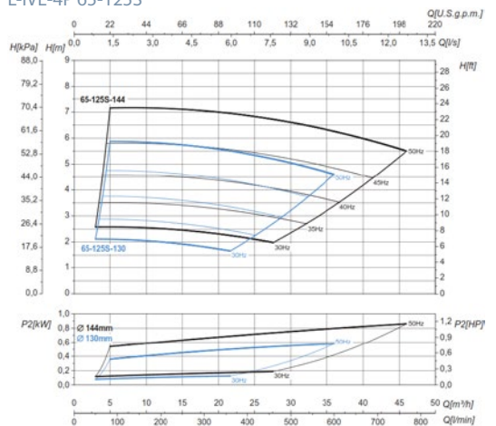
L-IVE-4P 65-125S
