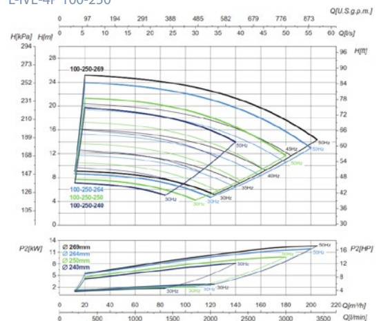
L-IVE-4P 100-250
