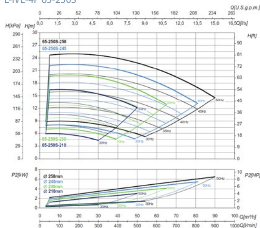
L-IVE-4P 65-250S
