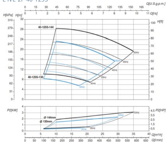
L-IVE-2P 40-125S
