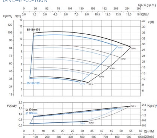
L-IVE-4P 65-160N
