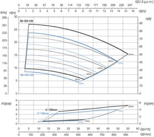
L-IVE-2P 50-125
