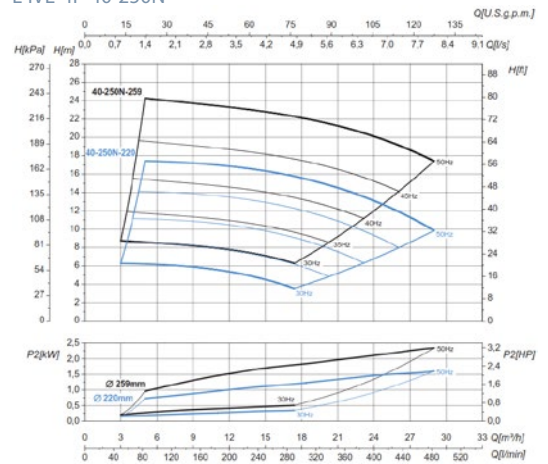
L-IVE-4P 40-250N
