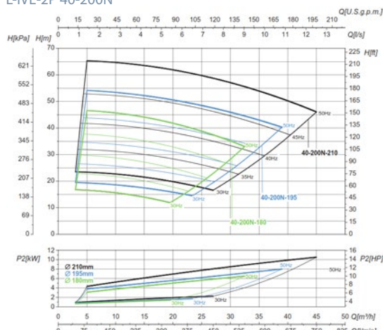
L-IVE-2P 40-200N
