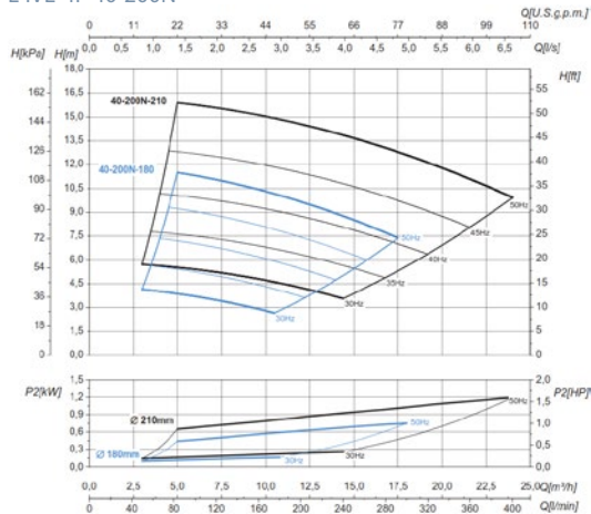
L-IVE-4P 40-200N
