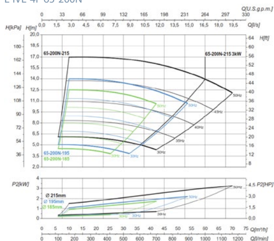
L-IVE-4P 65-200N
