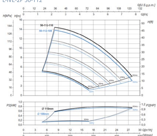
L-IVE-2P 50-112
